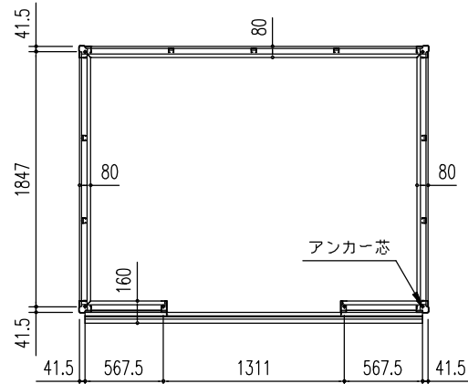
床 伏 図 (S = 1/50)
