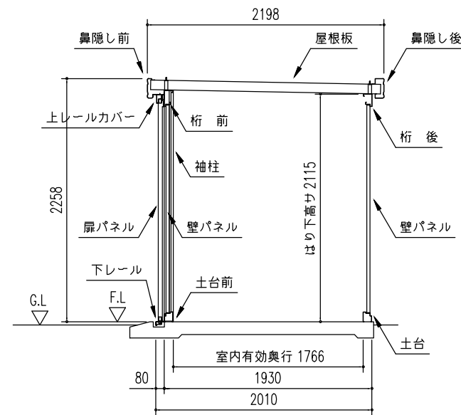
矩計図 (S = 1/50)
