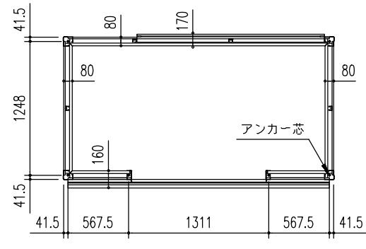
床 伏 図 (S = 1/50)
