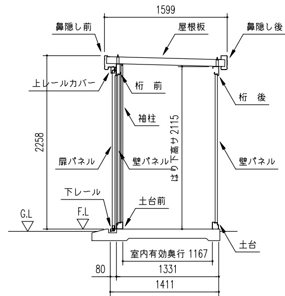
矩計図 (S=1/50)
