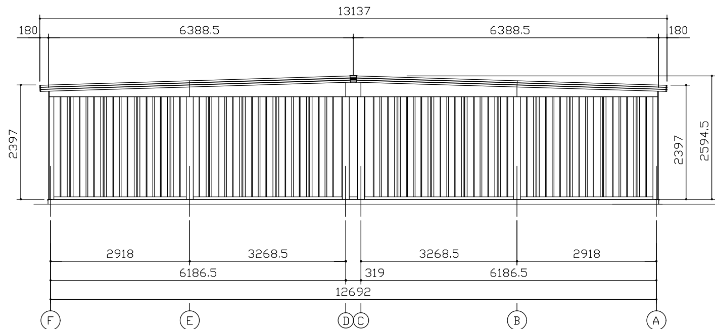
側面立面図 (S=1/80)
