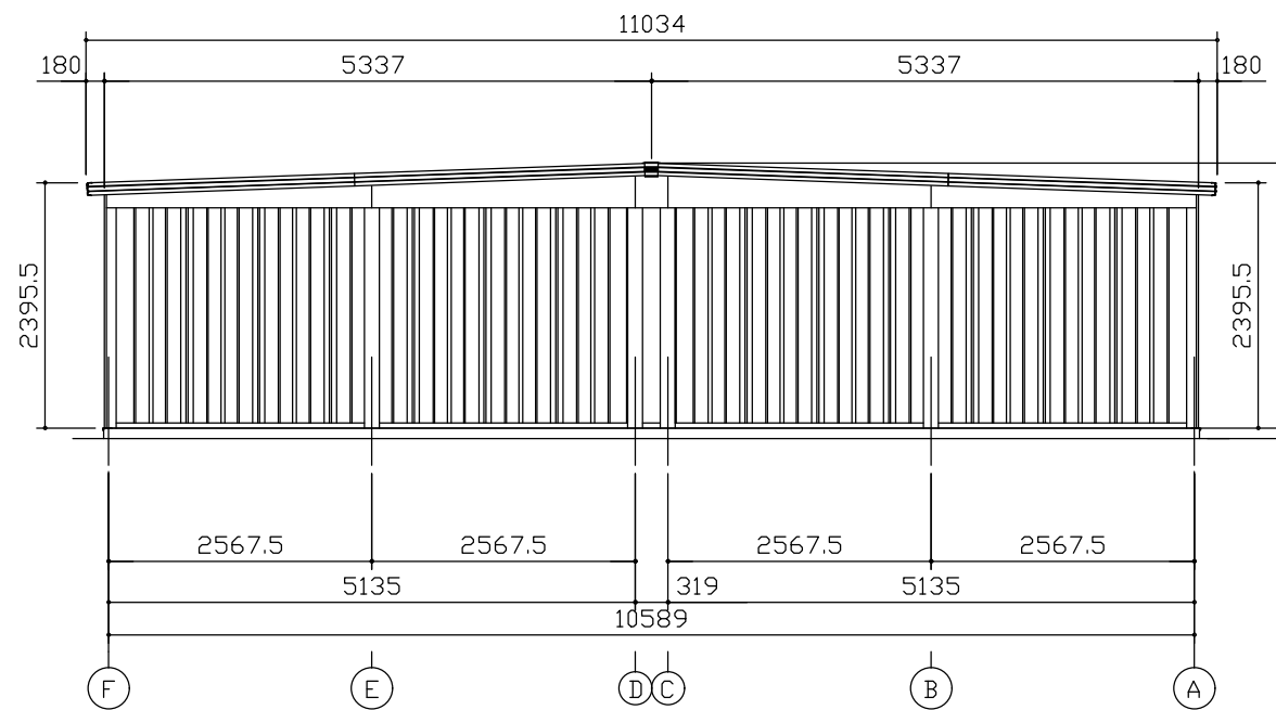
側面立面図 (S=1/80)
