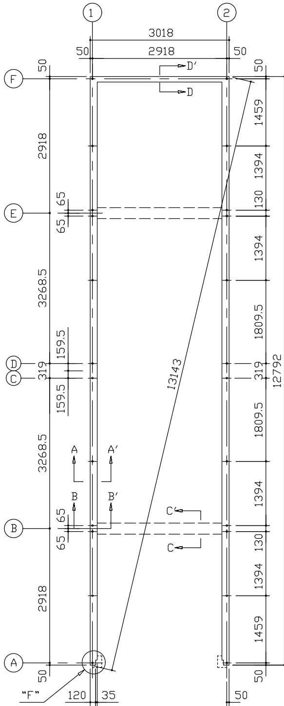
布基礎伏図 (S=1/80)
