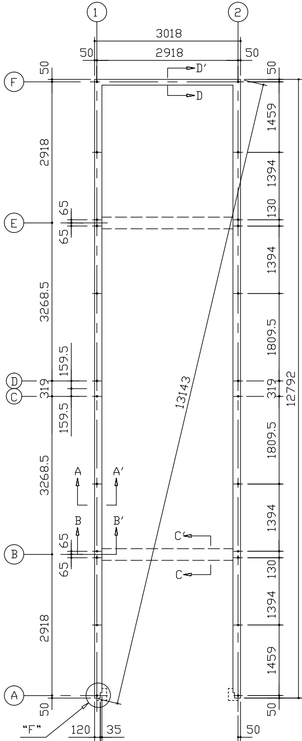
布 基 礎 伏 図 (S= 1/80)
