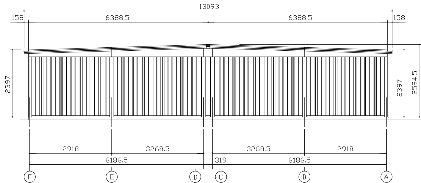
側面立面図 (S=1/80)
