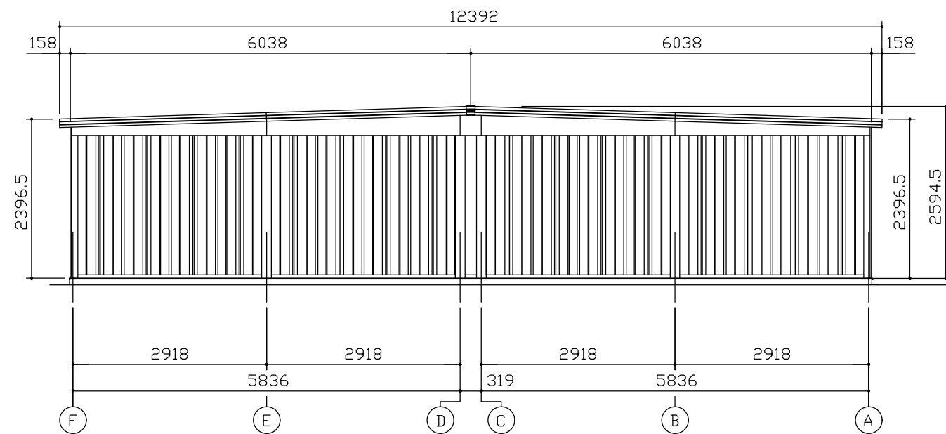
側面立面図 (S=1/80)
