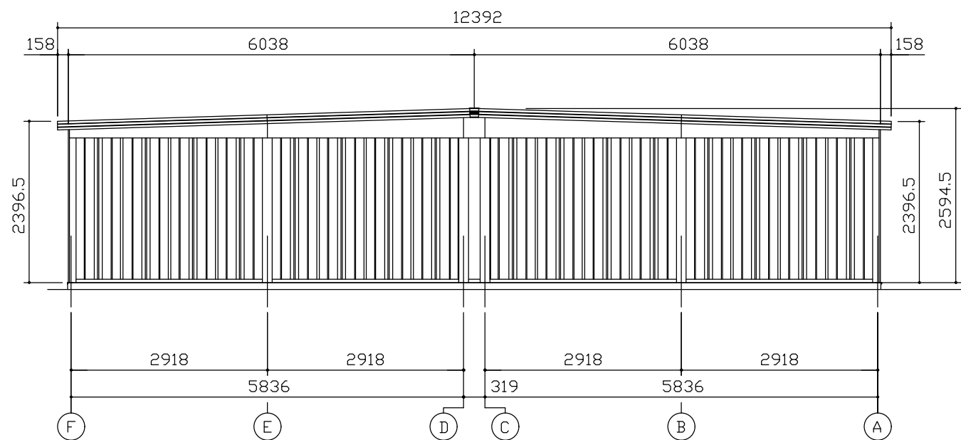
側面立面図 (S=1/80)
