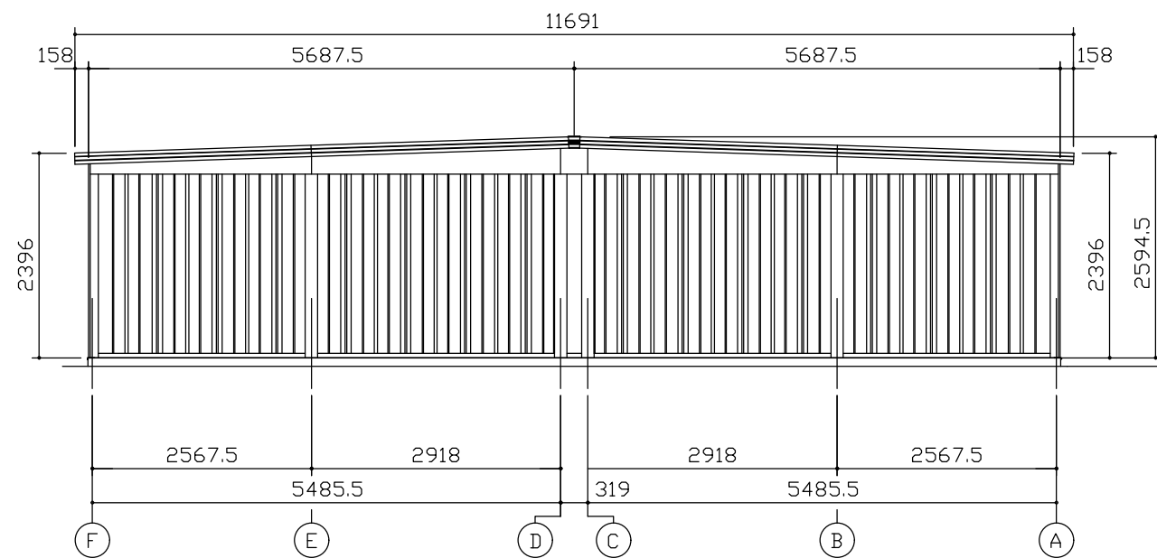
側面立面図 (S=1/80)
