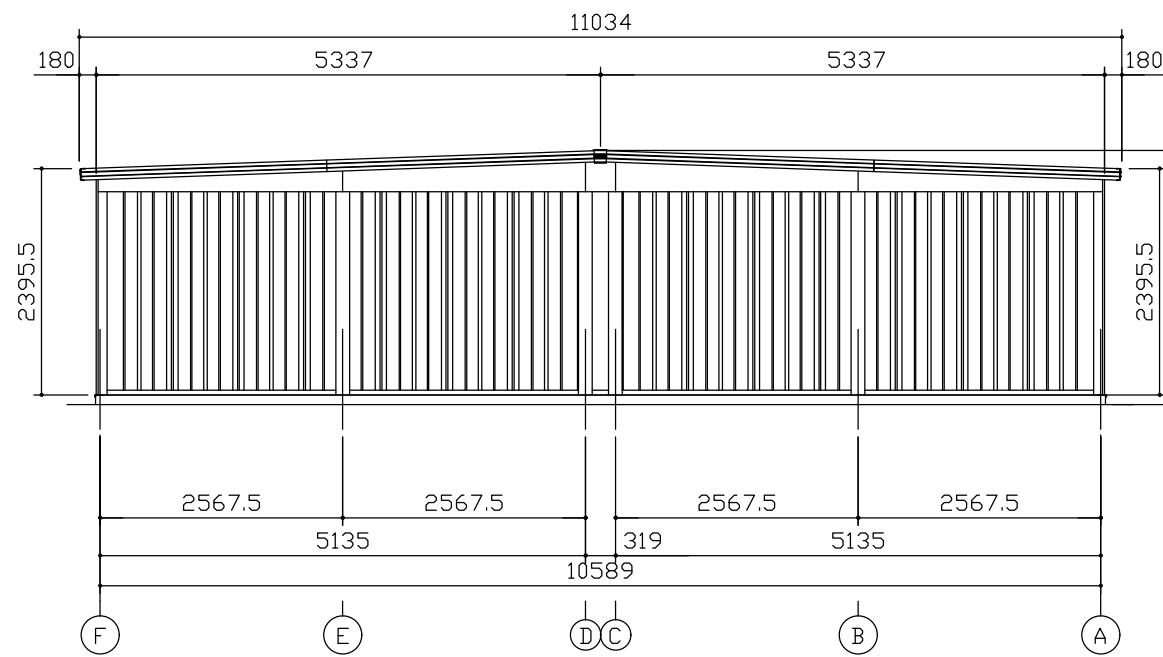
側面立面図 (S=1/80)
