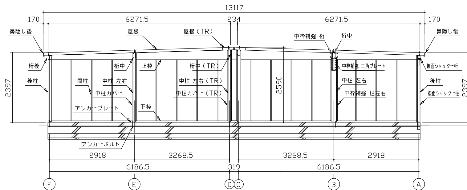
側面断面図 (S=1/80)
