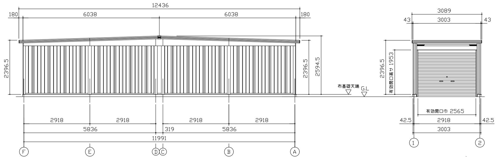
正面立面図 (S=1/80)
