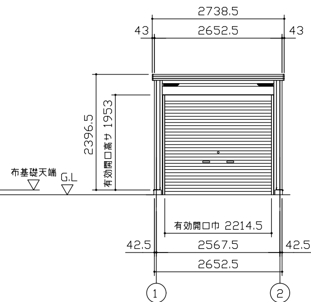
正面立面図 (S=1/80)
