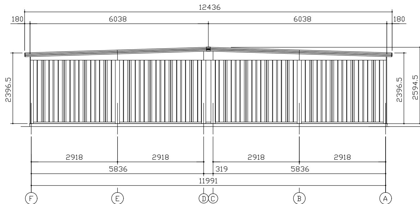
側面立面図 (S=1/80)
