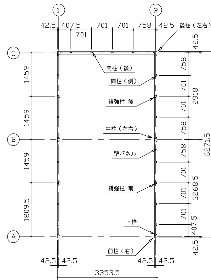
平面図 (S=1/80)
