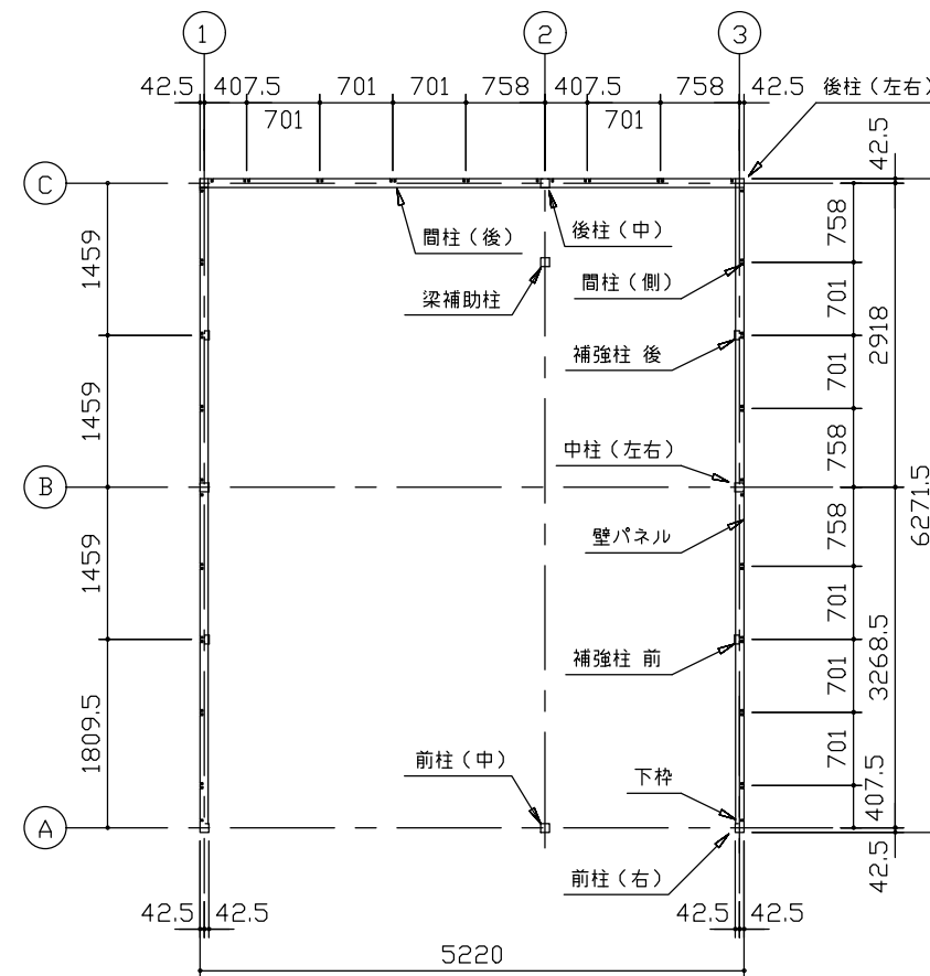
平面図 (S=1/80)
