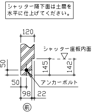
シャッター部分詳細図 ( S = 1/20 )
