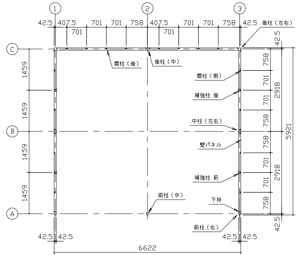
平面図 (S=1/80)
