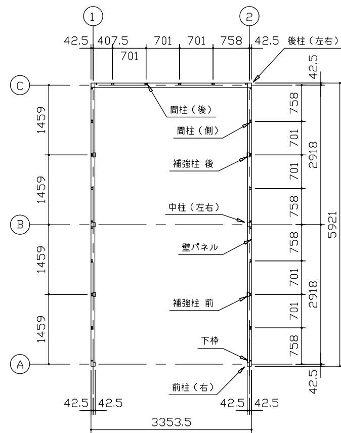
平面図 (S=1/80)
