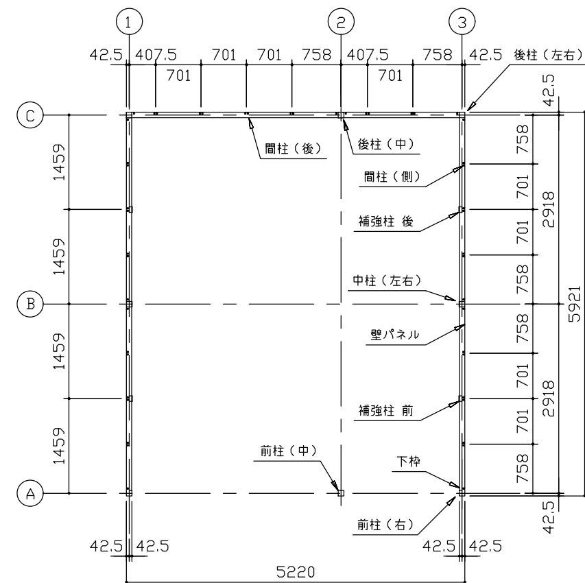
平面図 (S=1/80)
