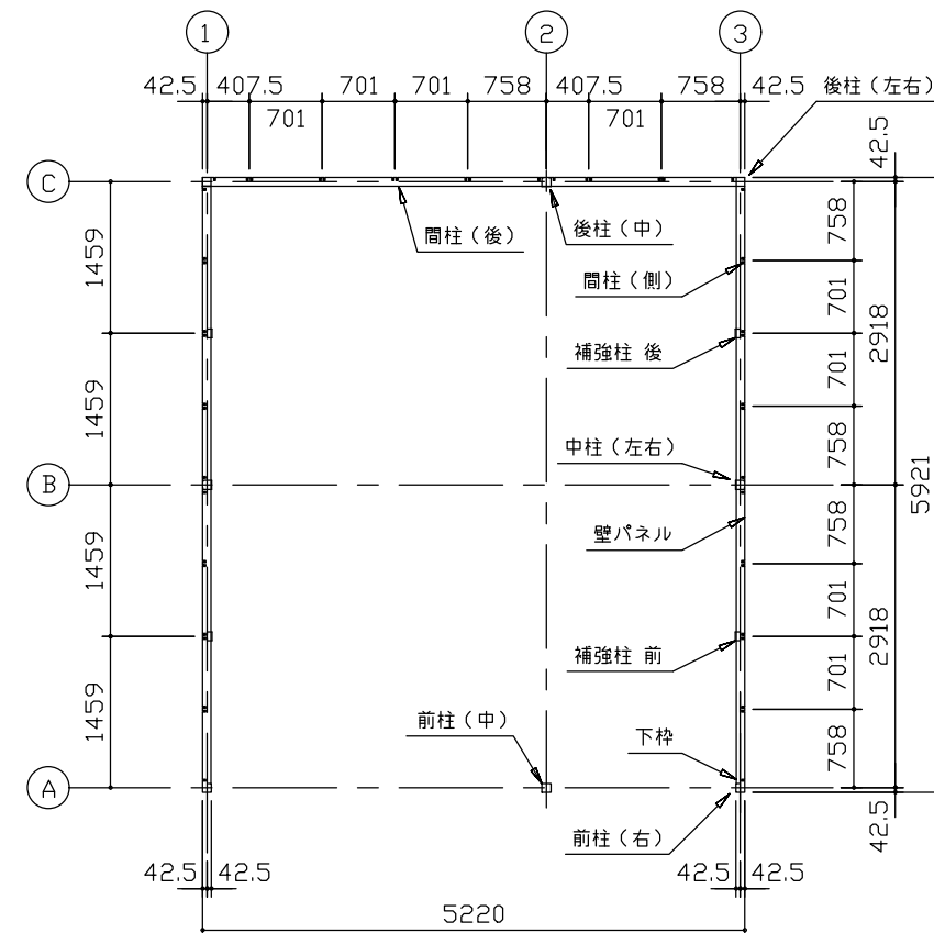
平面図 (S=1/80)
