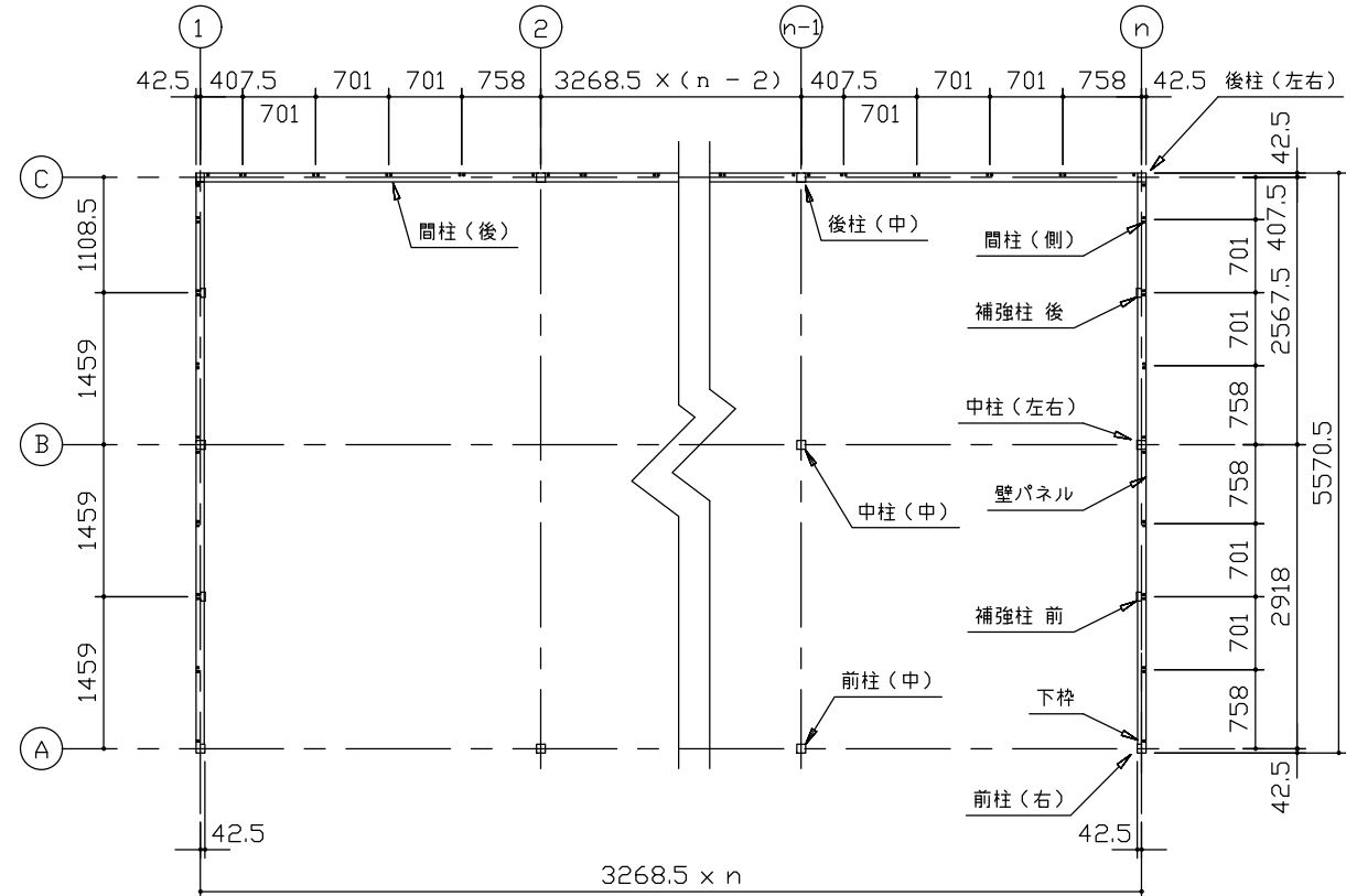
平面図 (S=1/80)
