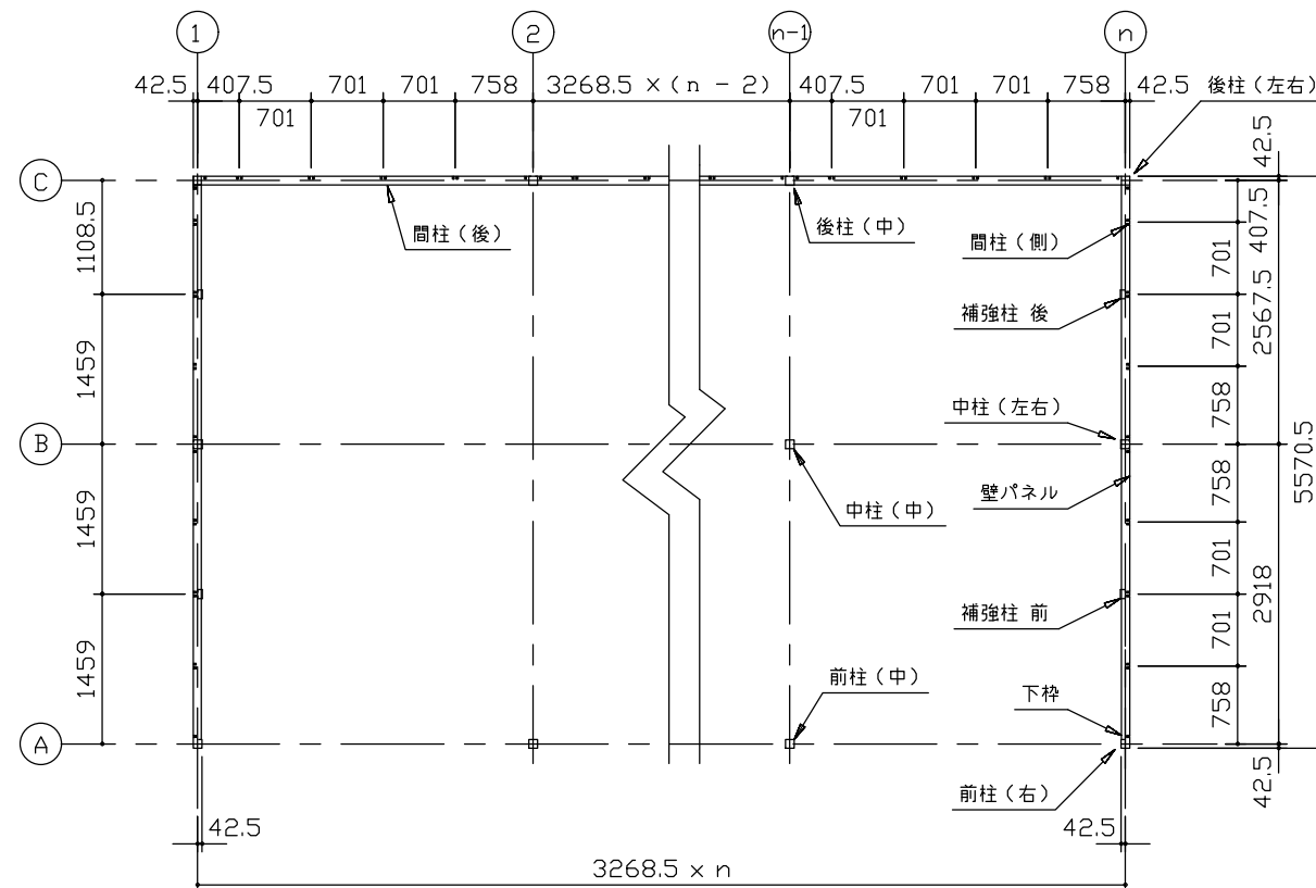
平面図 (S=1/80)
