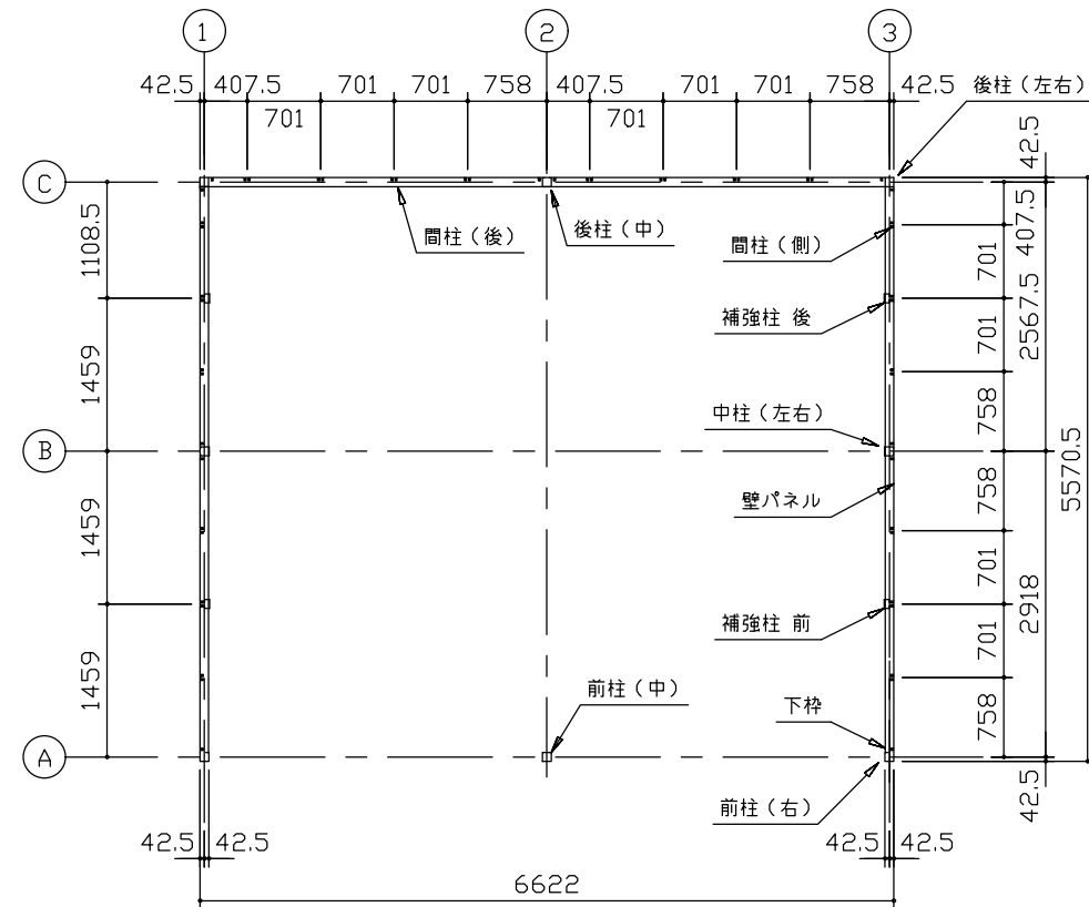
平面図 (S=1/80)
