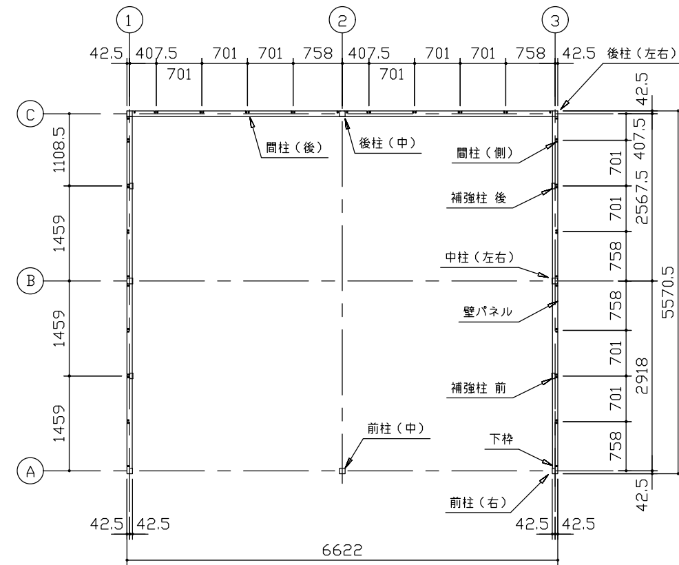
平面図 (S=1/80)
