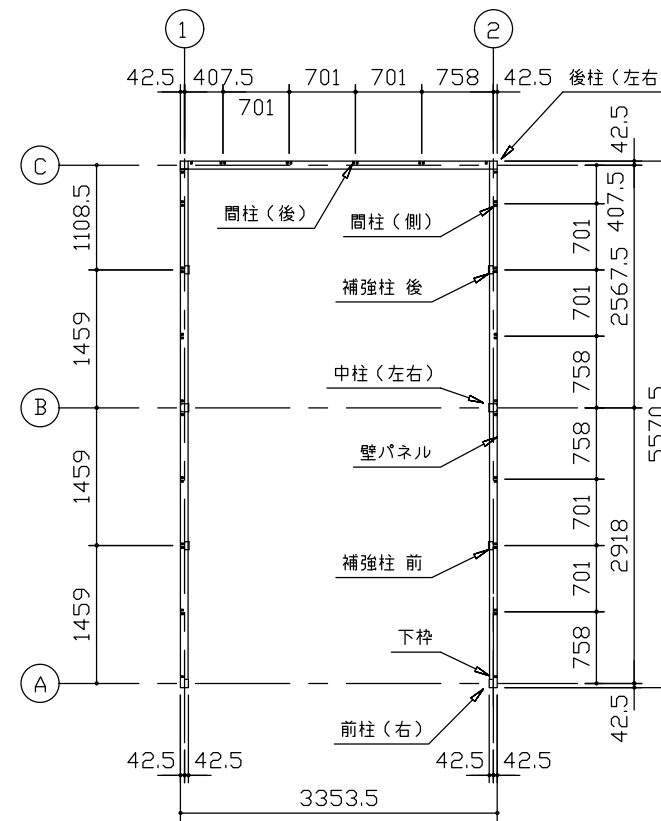
平面図 (S=1/80)
