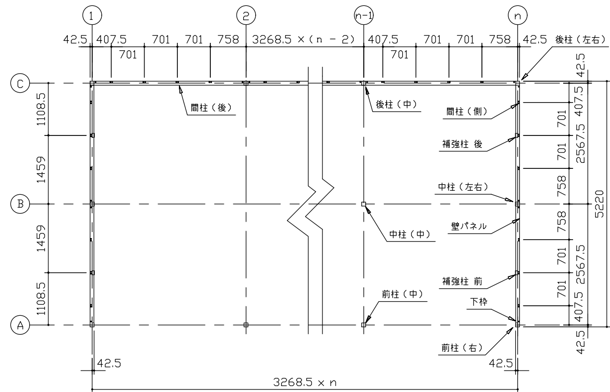
平面図 (S=1/80)
