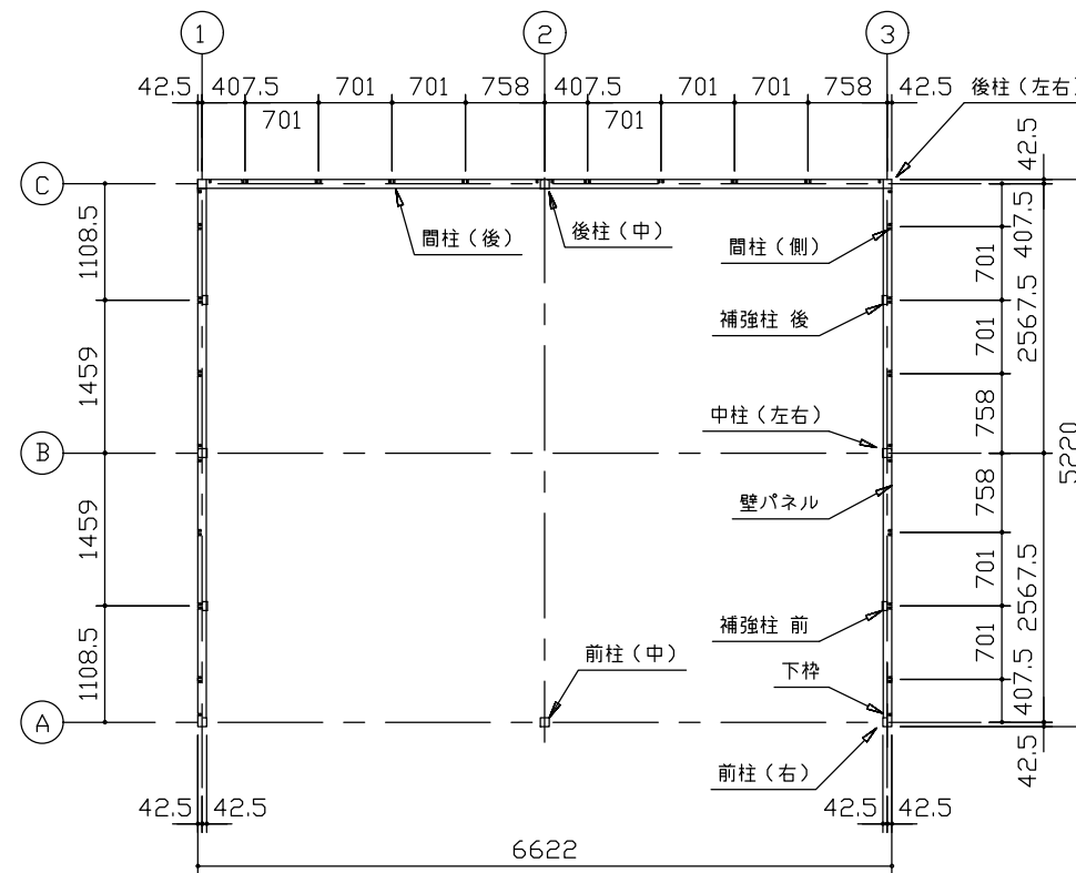
平面図 (S=1/80)
