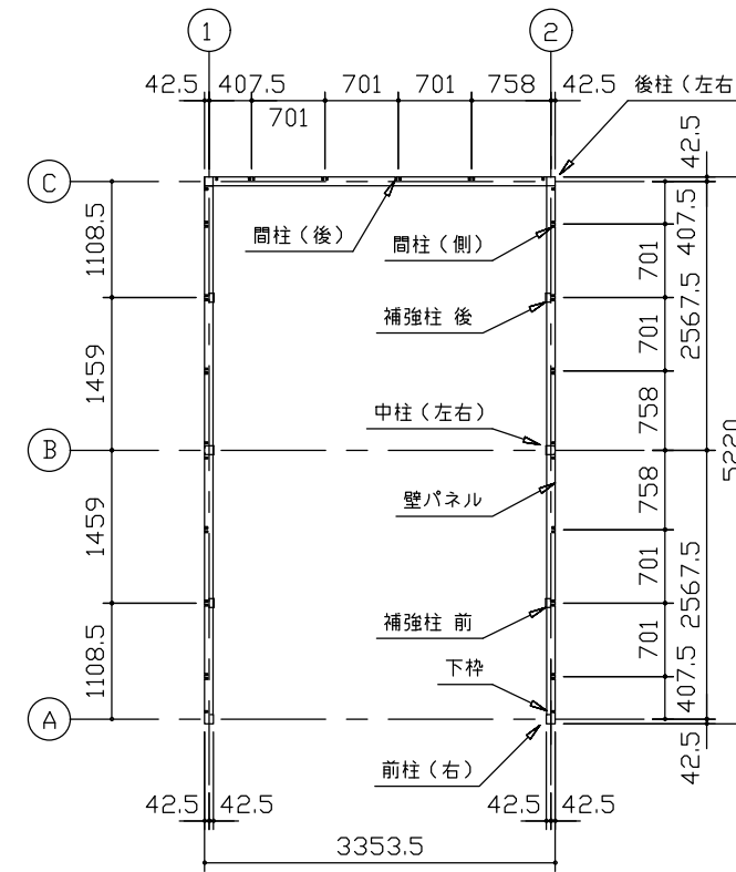
平面図 (S=1/80)
