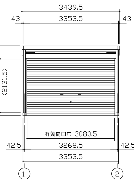
正面立面図 (S=1/80)
