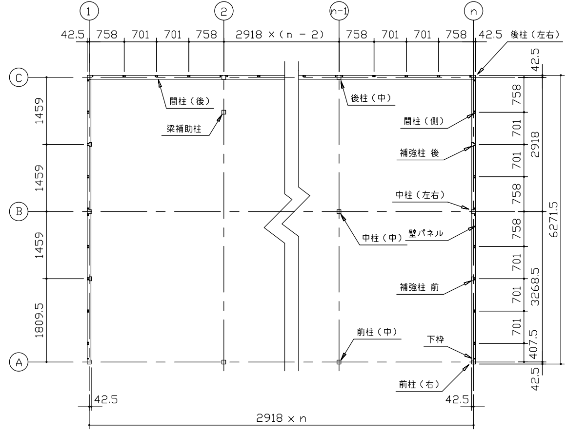
平面図 (S=1/80)
