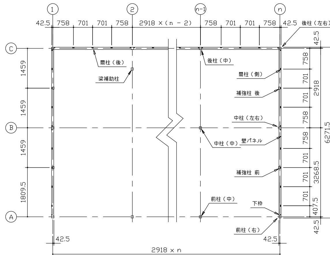
平面図 (S=1/80)
