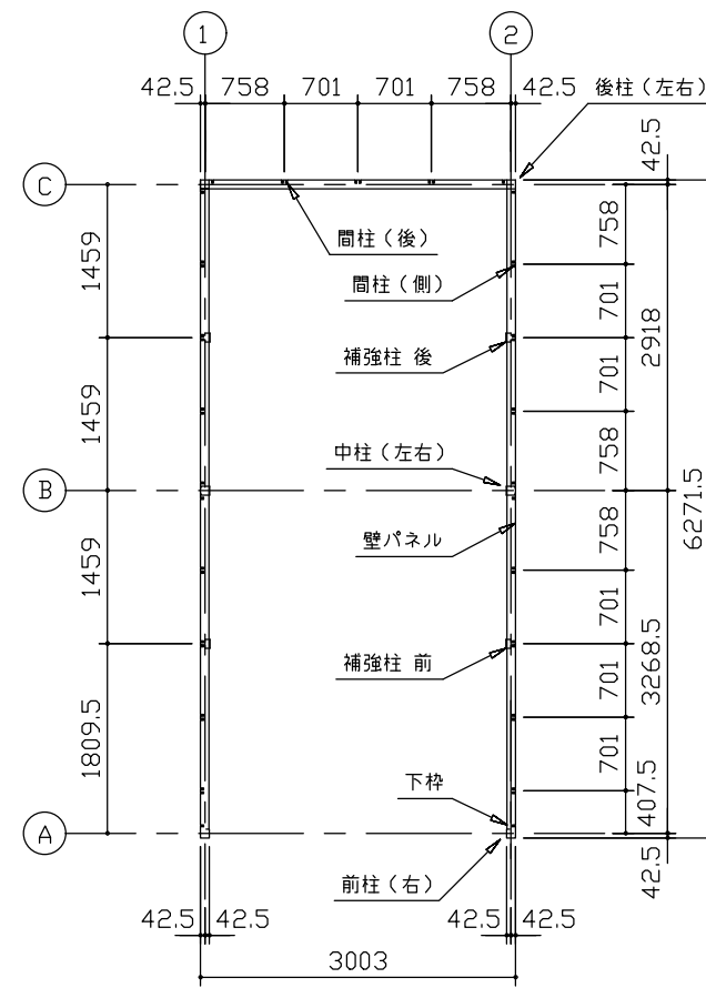
平面図 (S=1/80)
