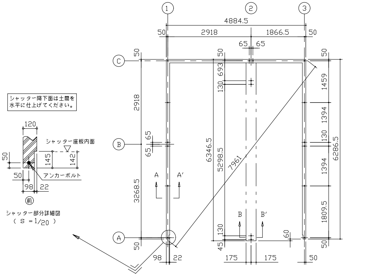
布 基 礎 伏 図 (S=1/80)
