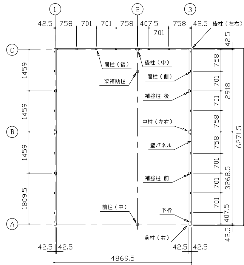
平面図 (S=1/80)
