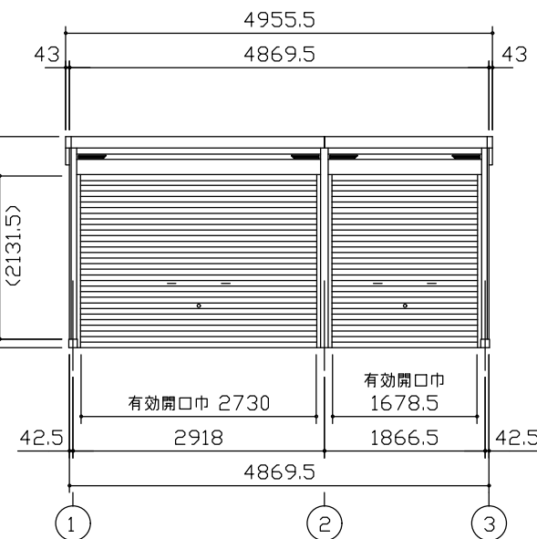
正面立面図 (S=1/80)
