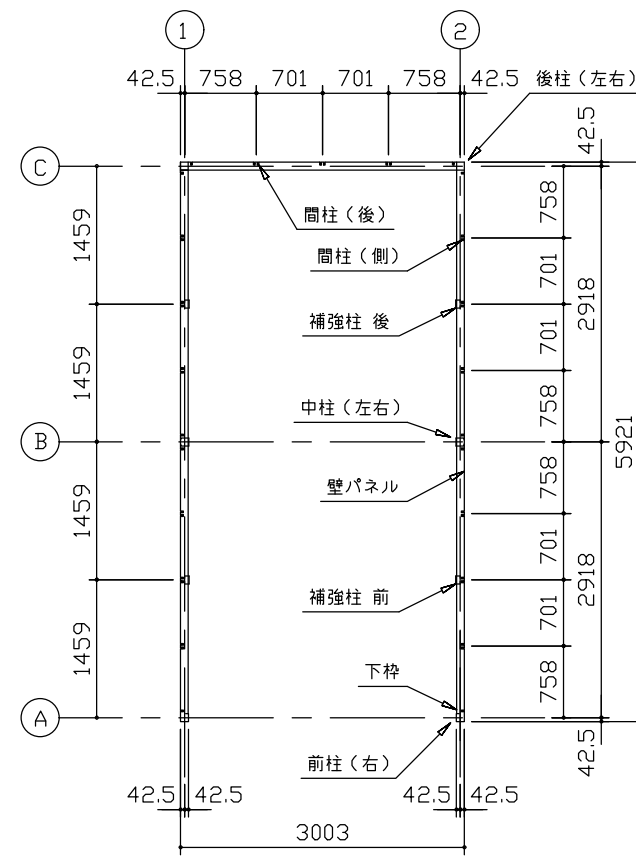
平面図 (S=1/80)
