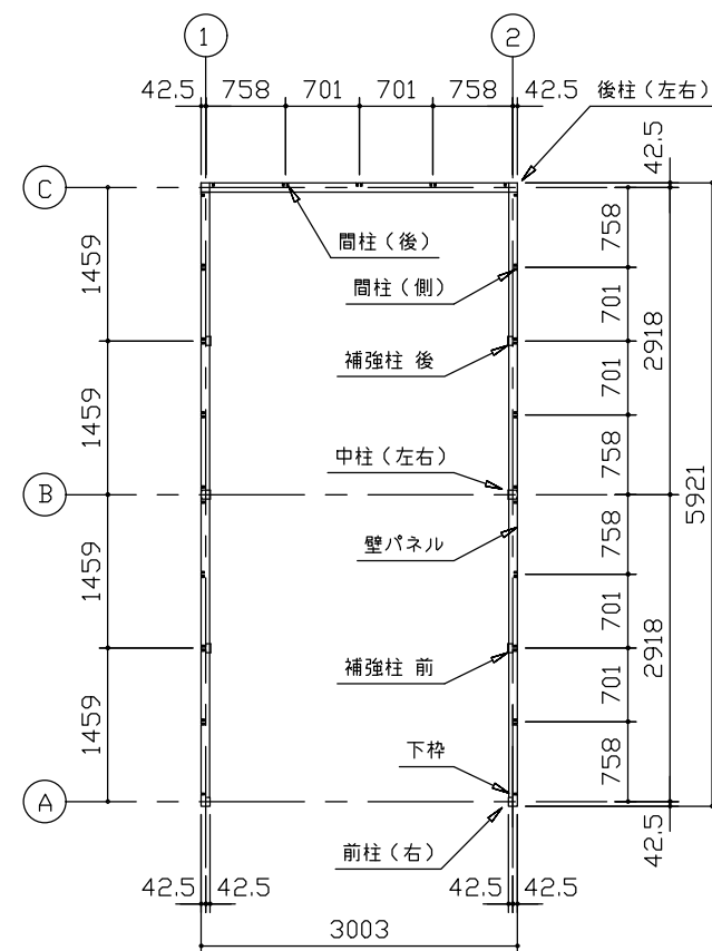
平面図 (S=1/80)
