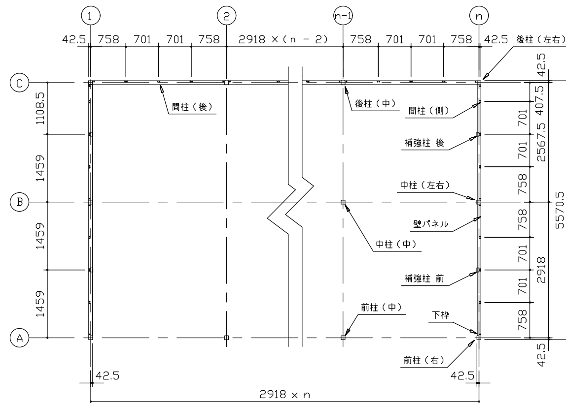
平面図 (S=1/80)
