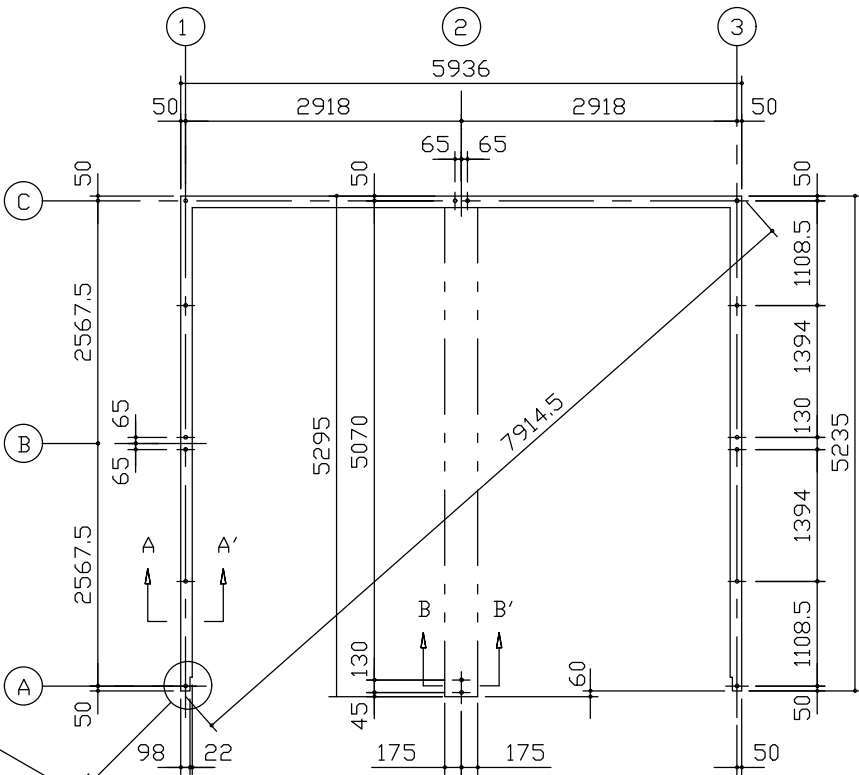
布 基 礎 伏 図 (S=1/80)
