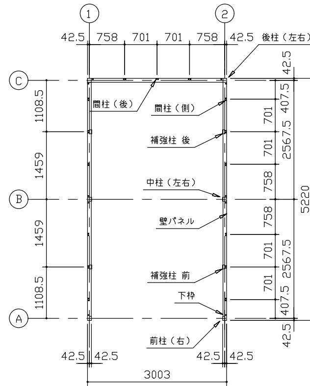
平面図 (S=1/80)
