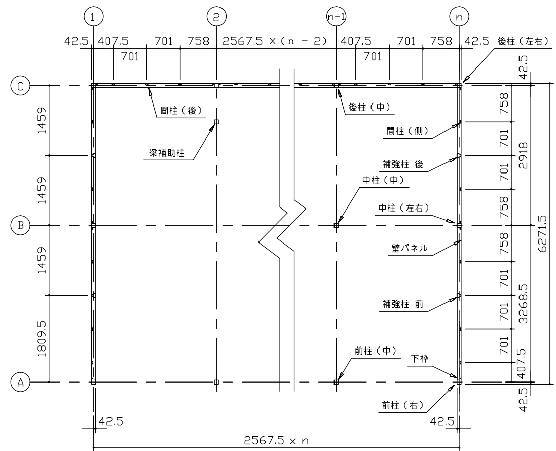
平面図 (S=1/80)
