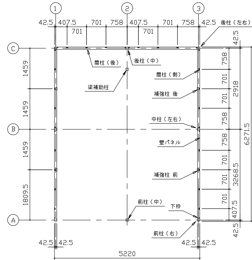
平面図 (S=1/80)
