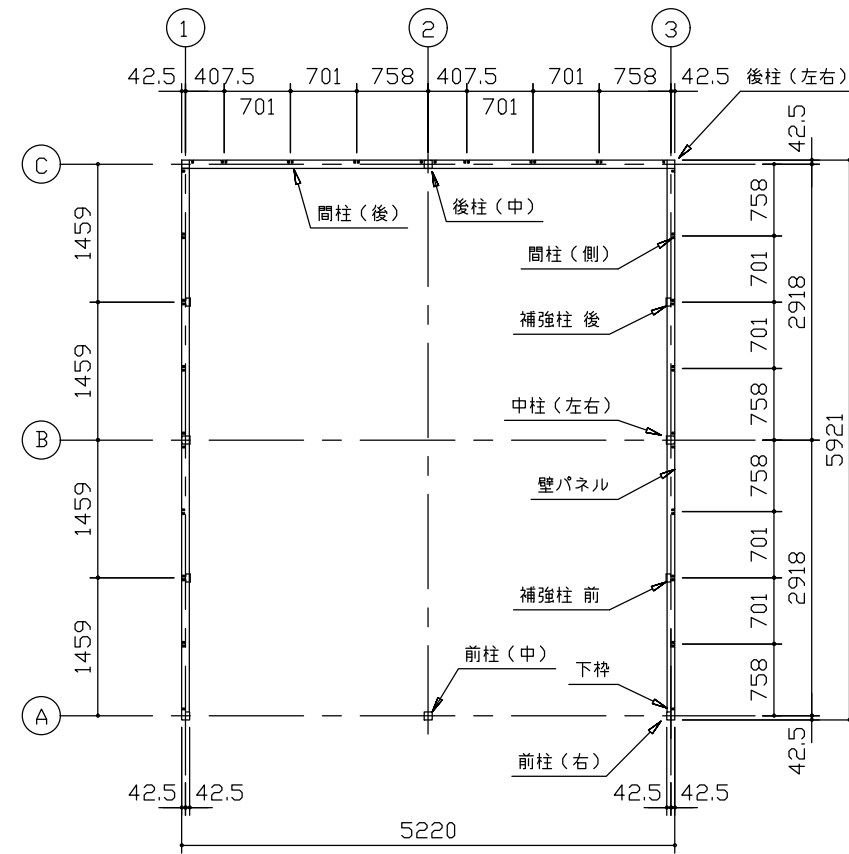
平面図 (S=1/80)
