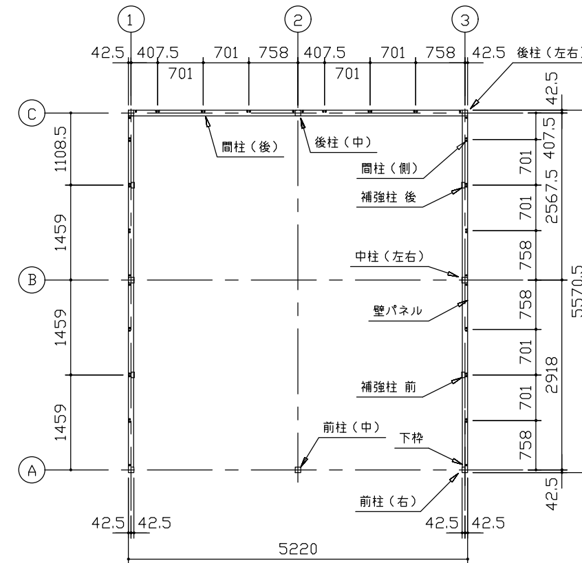
平面図 (S=1/80)
