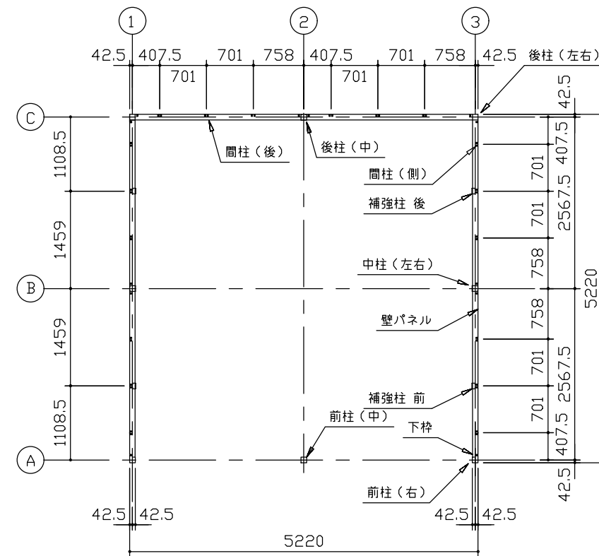
平面図 (S=1/80)
