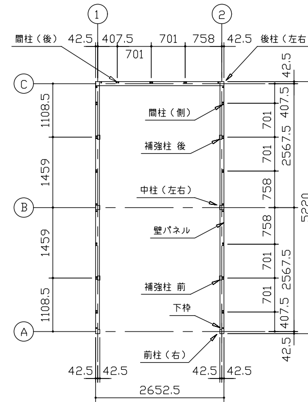
平面図 (S=1/80)
