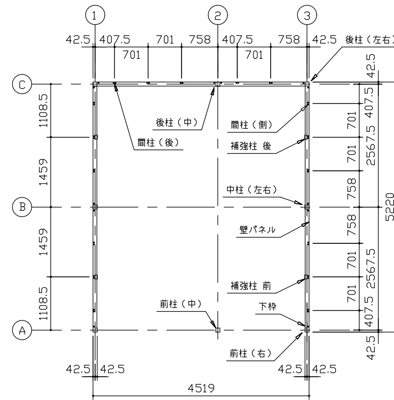
平面図 (S=1/80)
