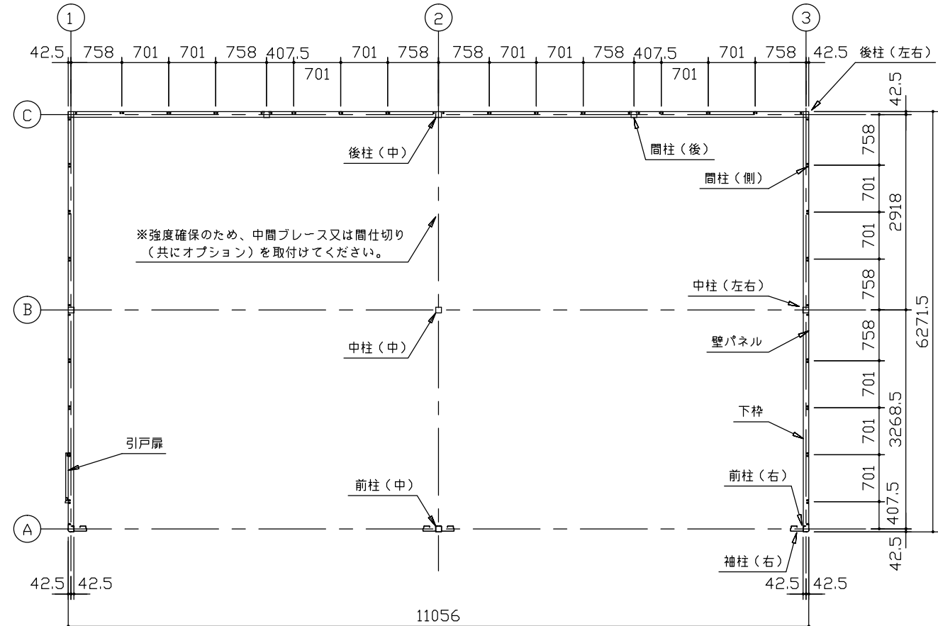
平面図 (S= 1/80)
