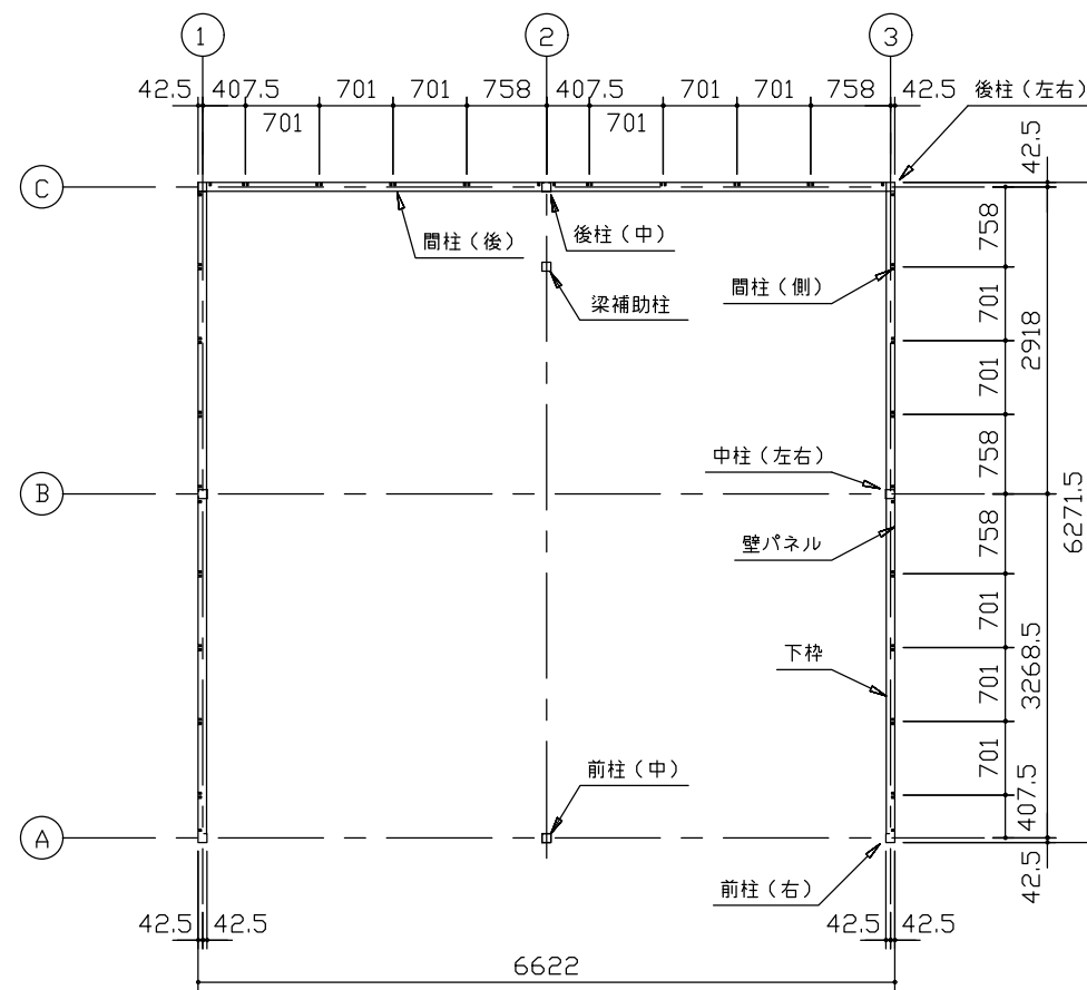
平面図 (S=1/80)
